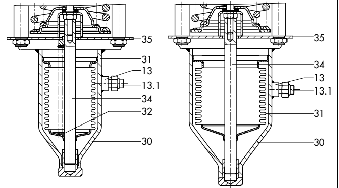
各种类型的 2413 型执行机构
