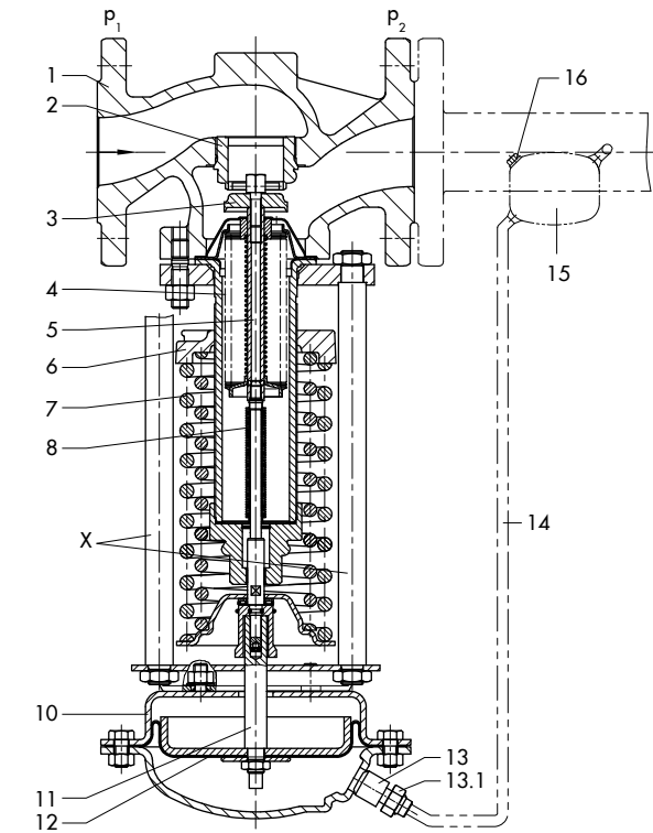
41-23 型通用减压阀剖面图
